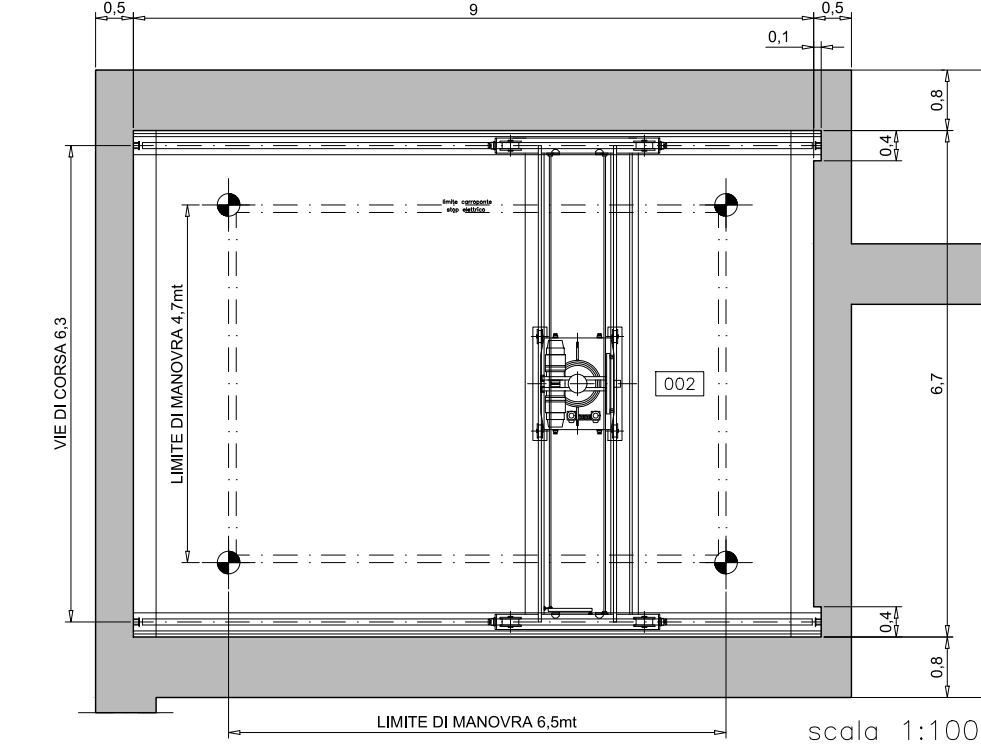
PIANTA CELLA A QUOTA +0.15
