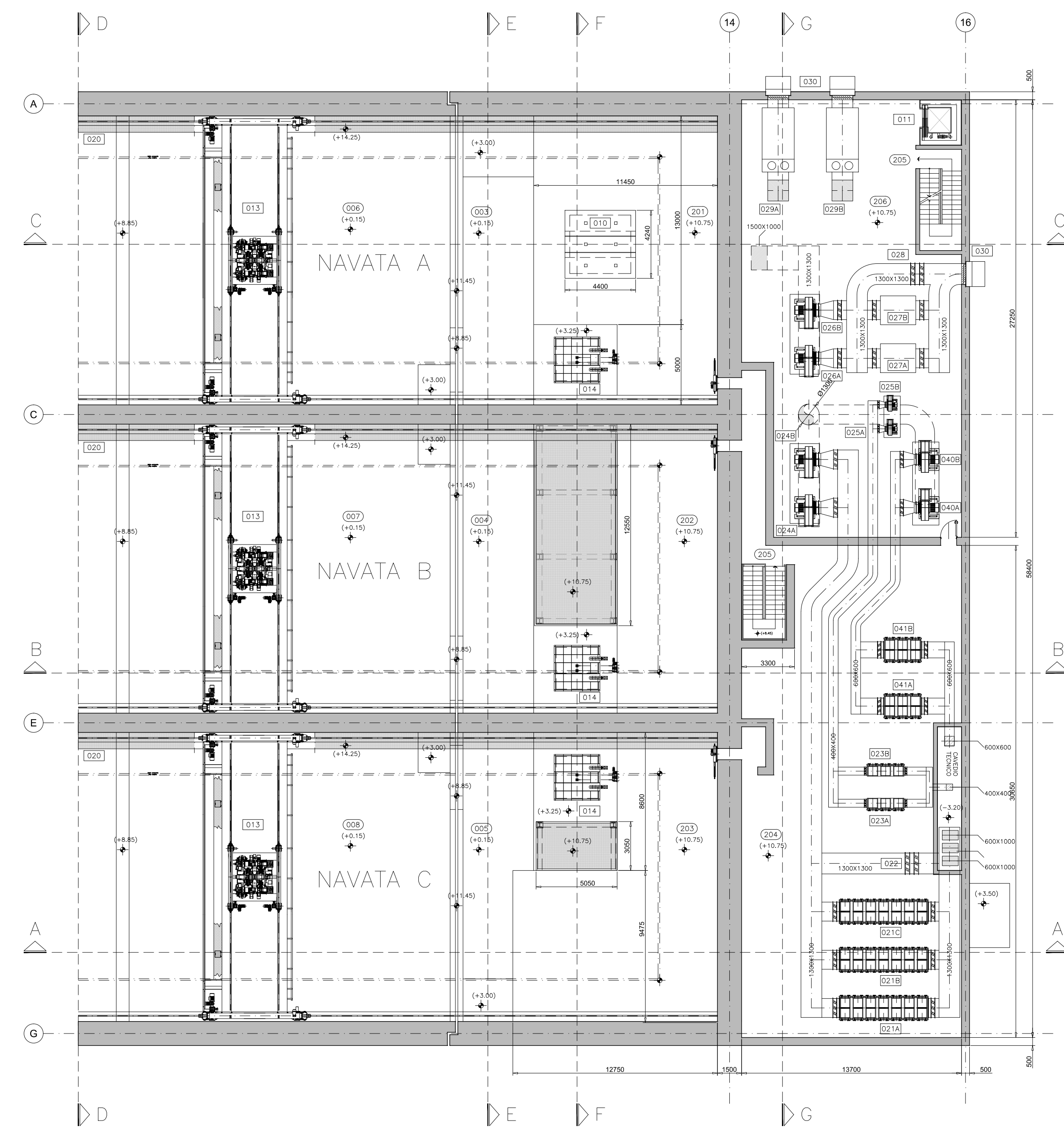
PIANTA PARZIALE PIANO SECONDO
