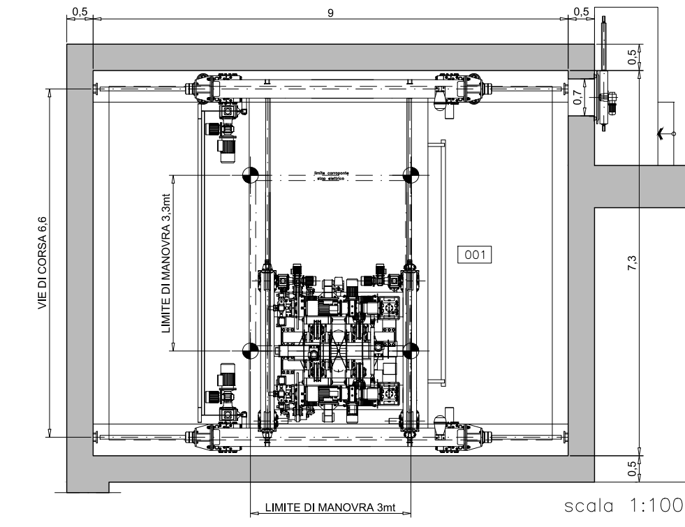
PIANTA CELLA A QUOTA +3.99
