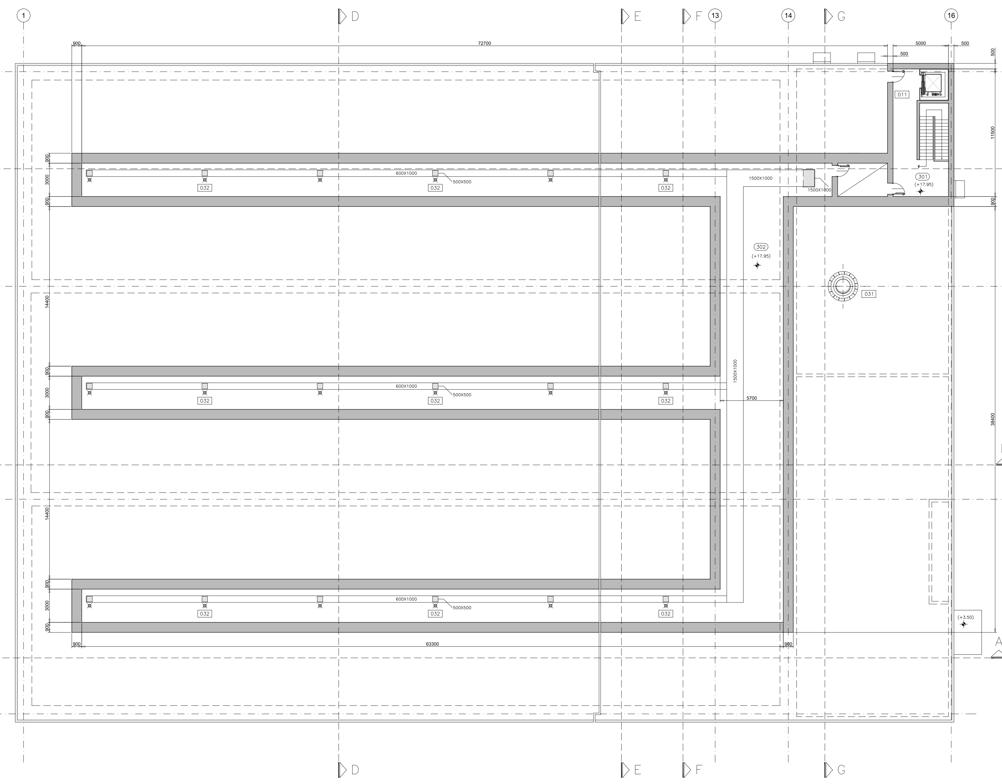
PIANTA PIANO COPERTURA
