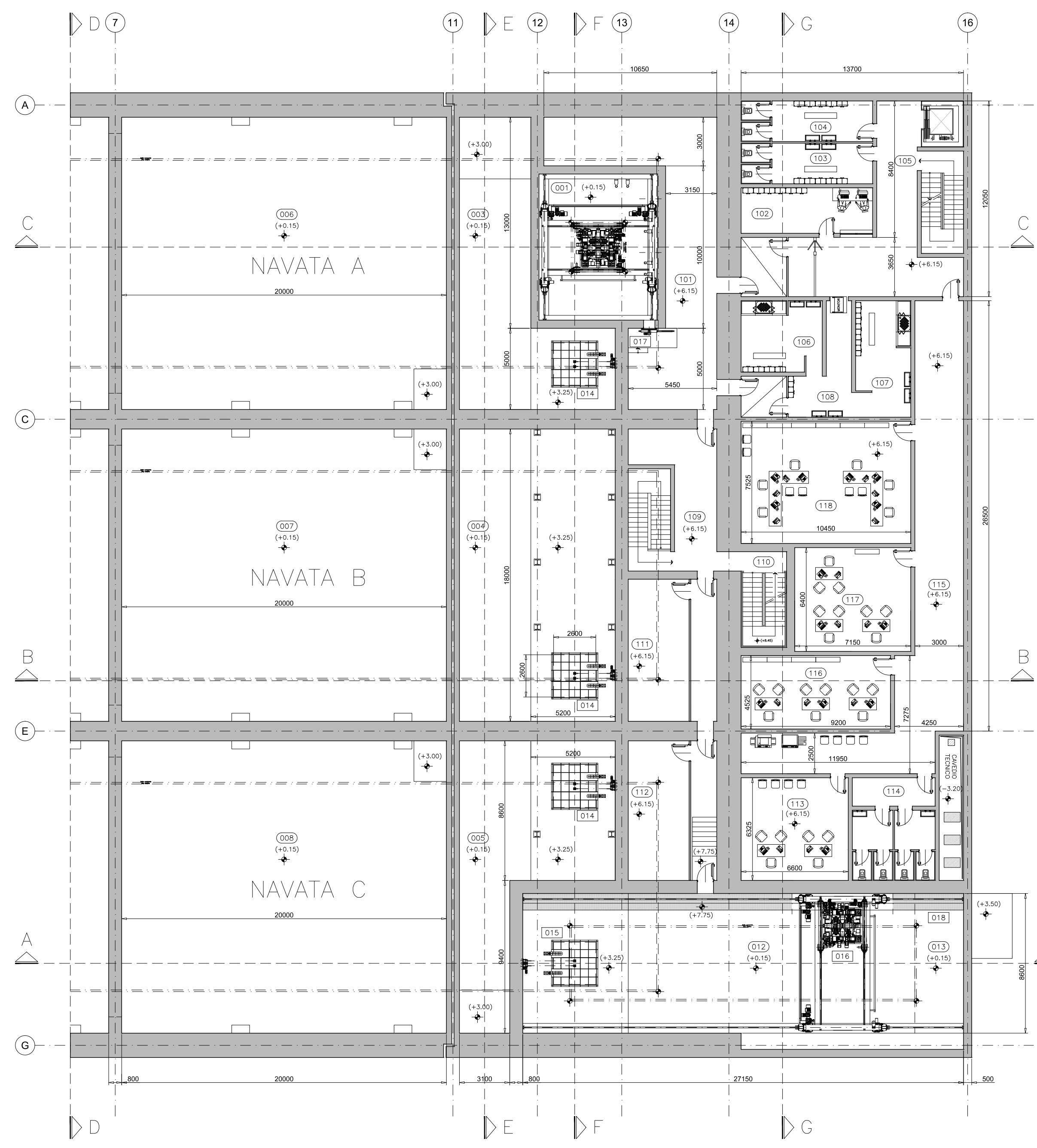
PIANTA PARZIALE PIANO PRIMO
