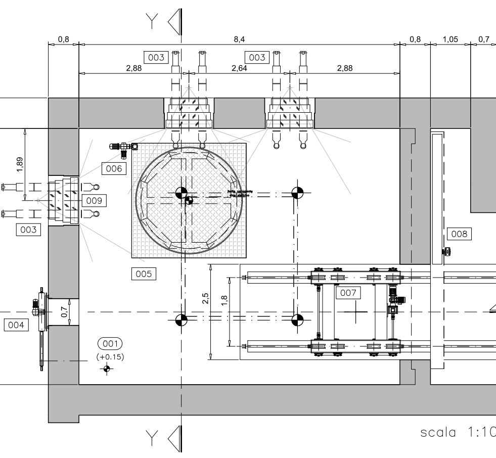
PIANTA CELLA A QUOTA +0.15
