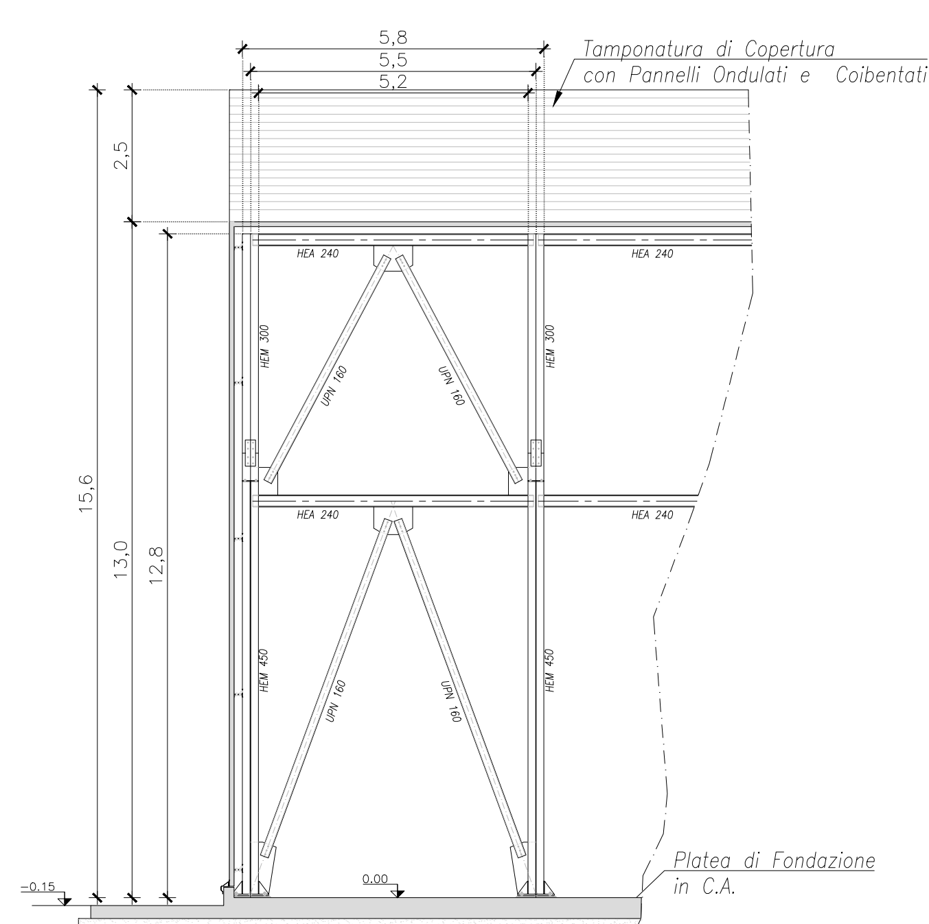
INDIVIDUAZIONE DIMENSIONI CARPENTERIA
