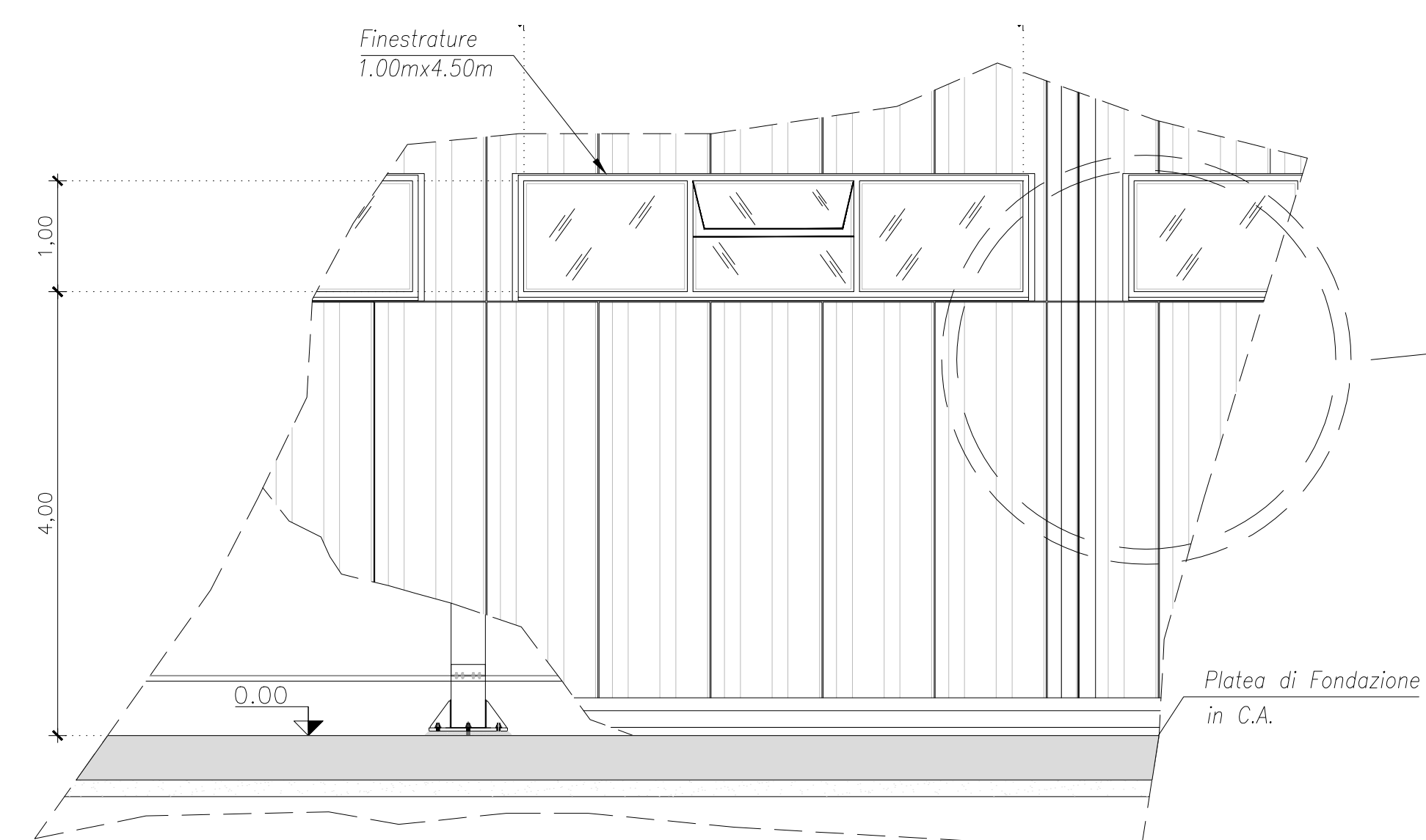
INDIVIDUAZIONE FINESTRATURE
