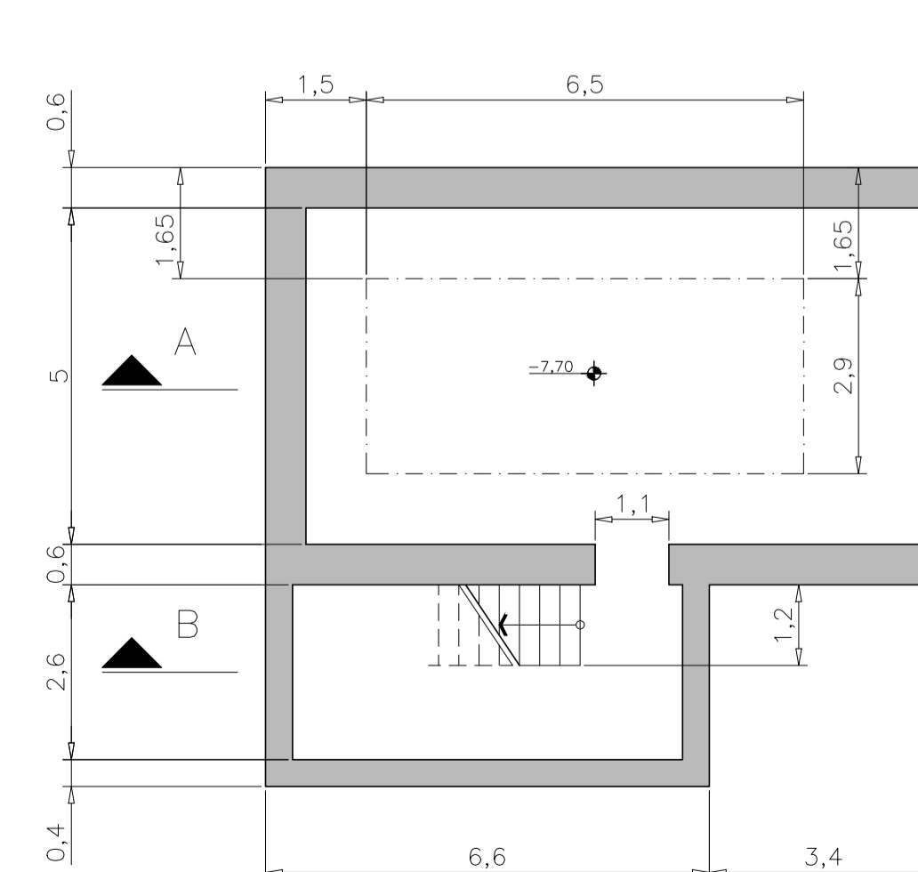
PIANTA A QUOTA -7,70 SCALA 1:100
