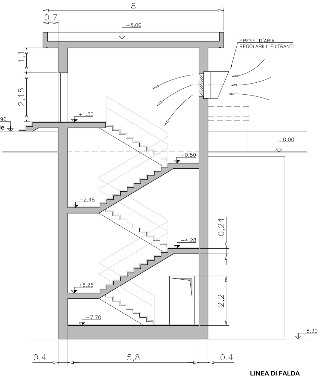
SEZIONE B-B SCALA 1:100
