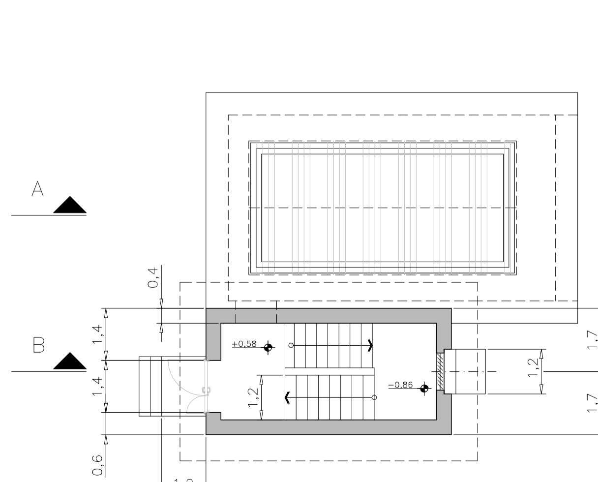
PIANTA A QUOTA +0,62 SCALA 1:100
