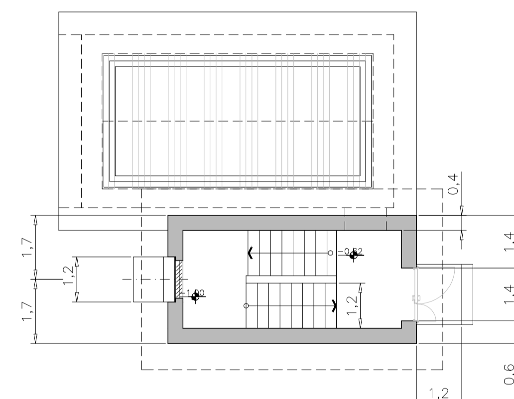
PIANTA A QUOTA +0,62 SCALA 1:100
