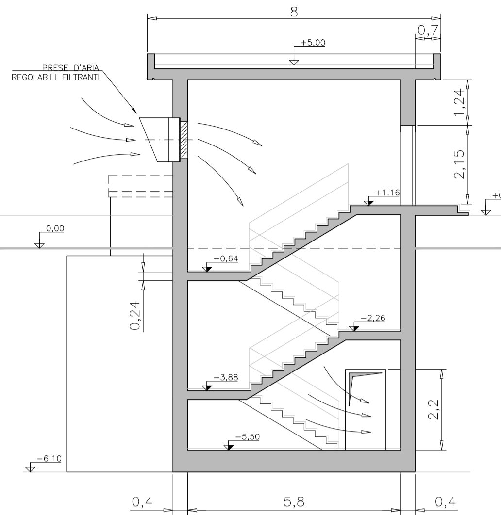
SEZIONE B-B SCALA 1:100
