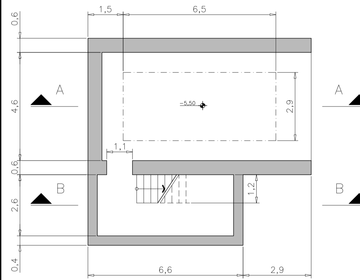
PIANTA A QUOTA -5,50 SCALA 1:100
